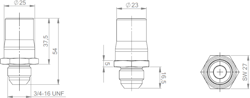
Coupler -08 Wig-200 compatible Z-Q 0200 0015
