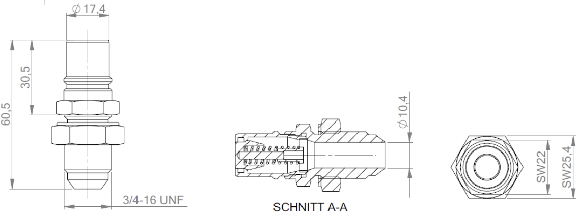
Nipple -08 Wig-200 compatible Z-Q 0200 0014
